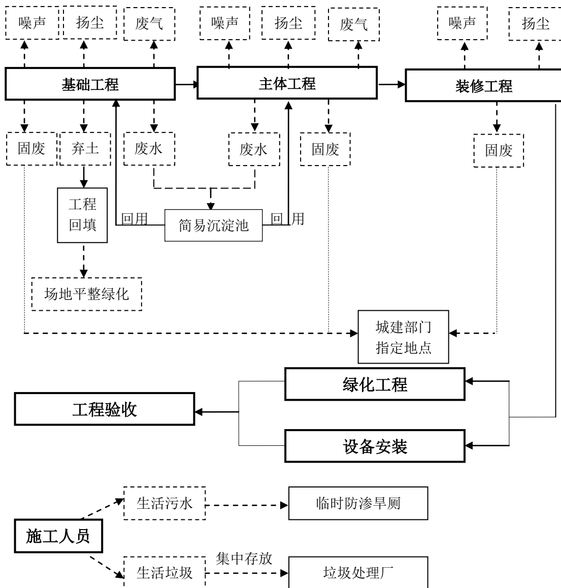
图 3 施工期工艺流程及污染物产生情况图
