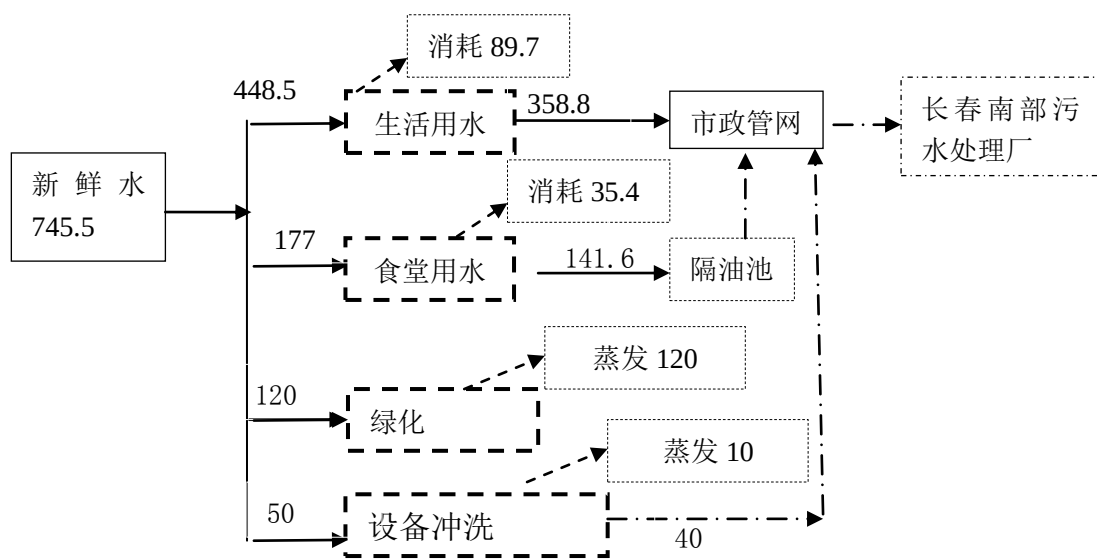
附图 2 项目水平衡图
