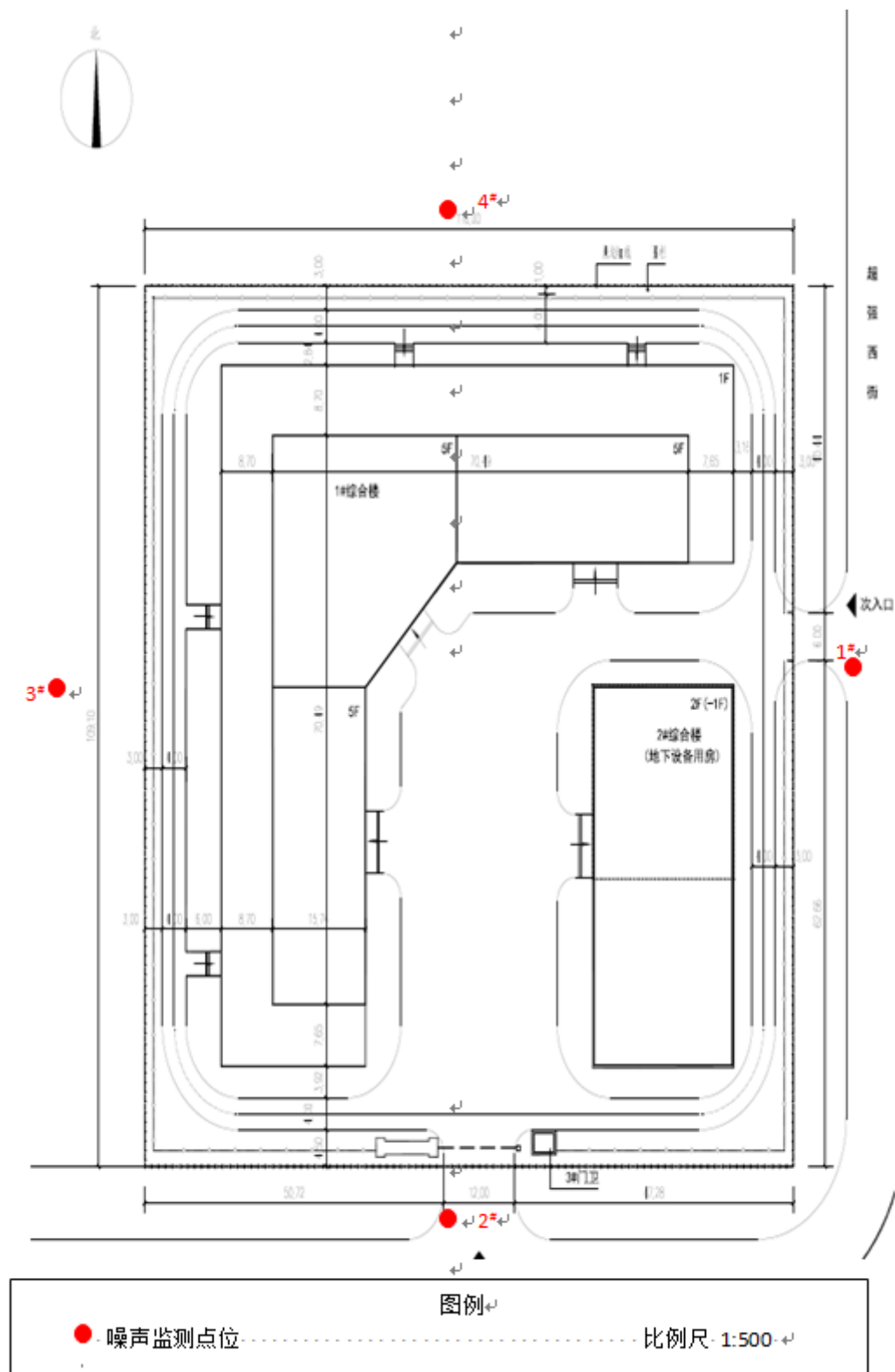
附图 3 项目厂区平面布置及噪声监测点位图
