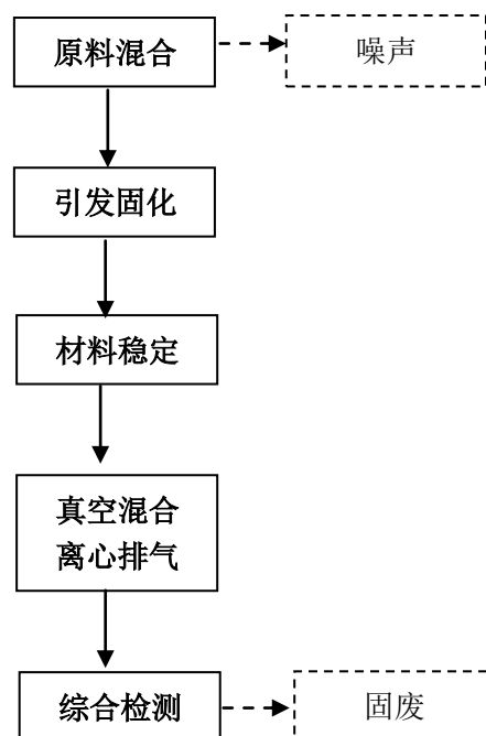
图 4 运营期工艺流程及污染物产生情况图
